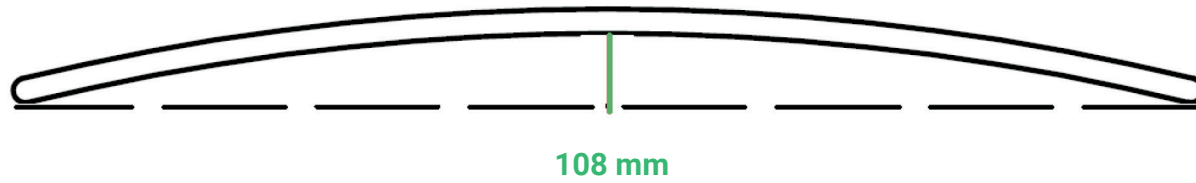
MAL HS. 67 • ENKELE BOCHT 1850 MM
