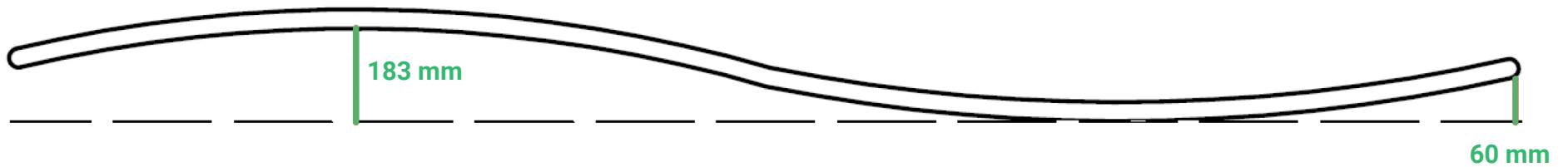
MAL HS. 8 + 250 MIDDEN • DUBBELE BOCHT 2900 MM
