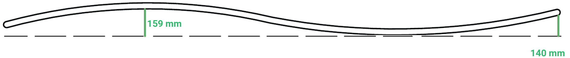
MAL HS. 8 + 750 MIDDEN • DUBBELE BOCHT 3500 MM
