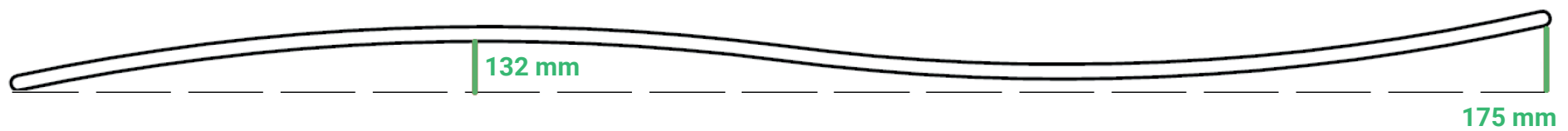
MAL HS. 55 + 500 MIDDEN • DUBBELE BOCHT 2950 MM
