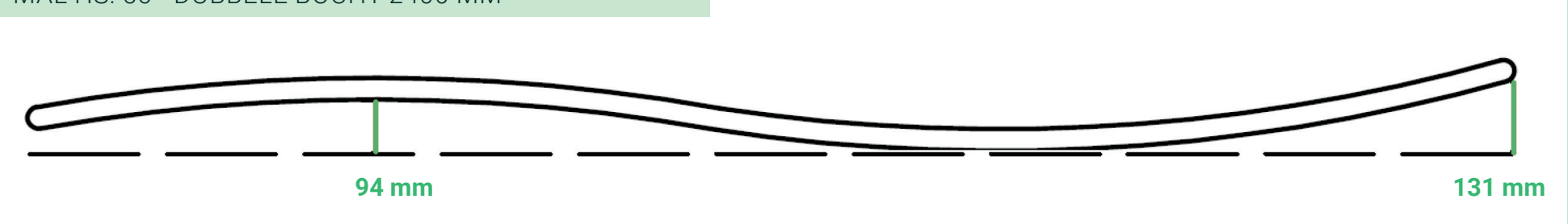
MAL HS. 56 • DUBBELE BOCHT 2400 MM
