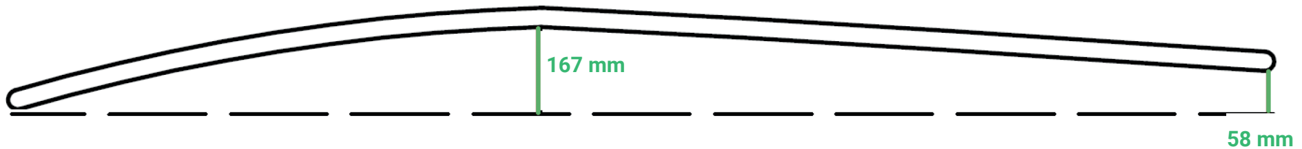
MAL HS. 49 • ENKELE BOCHT 2500 MM
